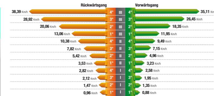
Grafische Darstellung der Geschwindigkeiten in Km/h - Betriebsdrehzahl Motor: 2800 Umdr./min.
